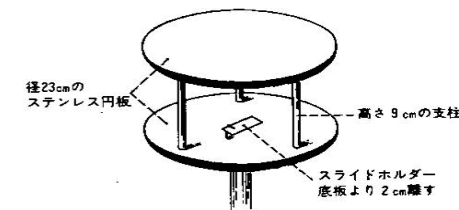
【↑花粉捕集器(ダラム型・重力法)】 環境省ホームページより
